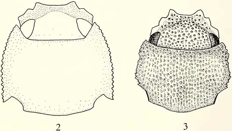
Abb. 2–3: Kopf und Halsschild von 2. Maechidius subcostatus Hell., 3. M. hirtipes Arr.
